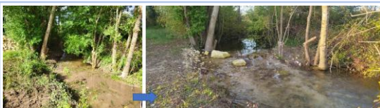
Recharge granulométrique par radiers sur le ruisseau des Jauges, affluent de l'Auge (1,5 km)
